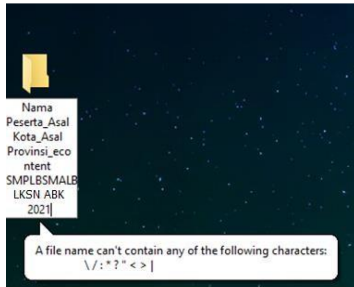
Gambar 1 : membuat folder
