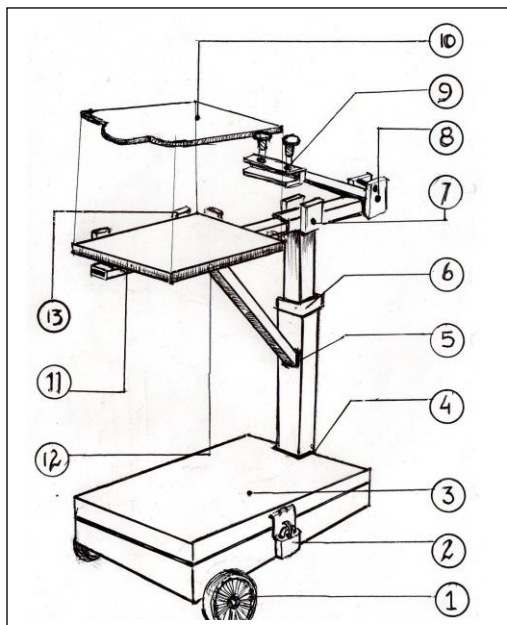
Gambar 4. Gambar Perspektif
