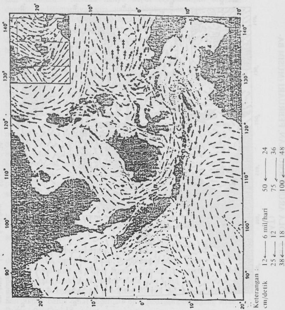
Peta 2 POLA ARUS PERMUKAAN (AGUSTUS), (MUSIM TI-MUR).
