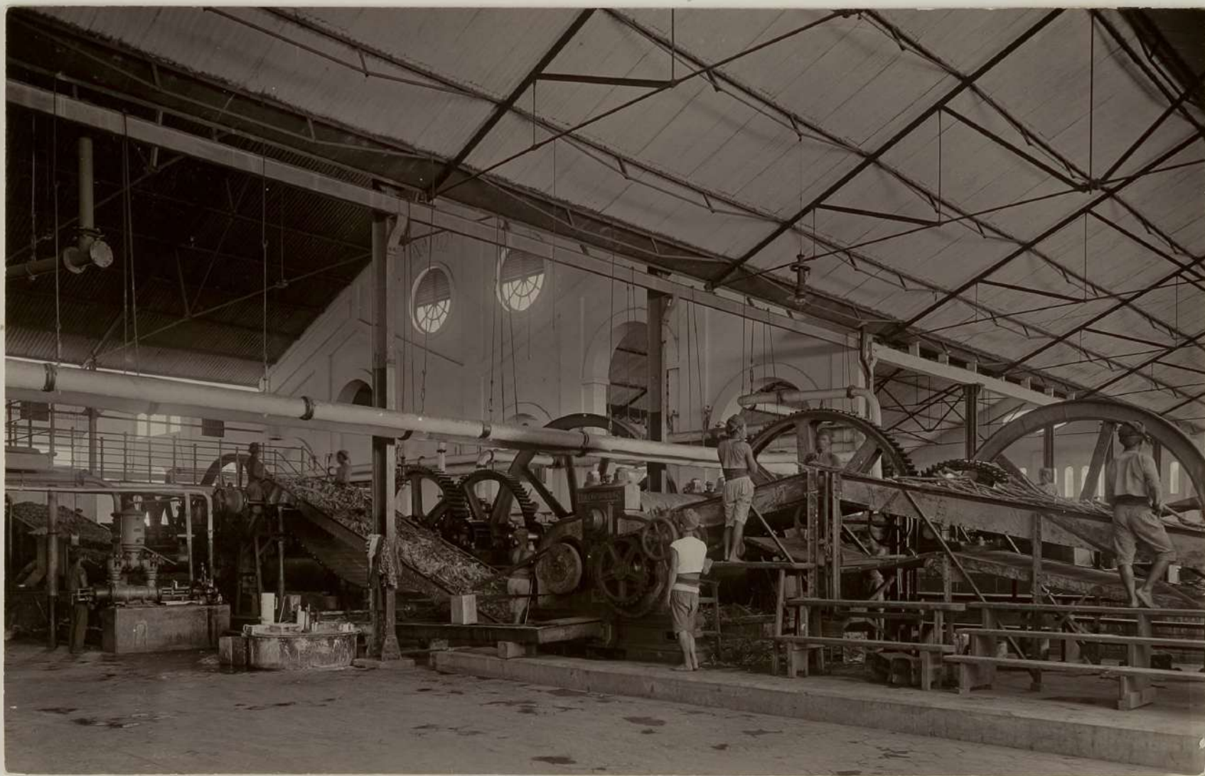
Gambar 3.6 Bagian dalam pabrik gula di Delanggu, sekitar tahun 1897. Sumber: Perpustakaan Universitas Leiden
