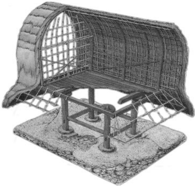
Gambar 15. Penampang Lumbung Suku Sasak (Sumber; www.wacana.co )
