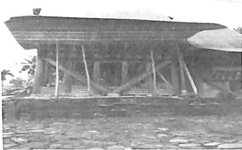
Tiang Rumah yang tinggi dan beralas batu pipih
