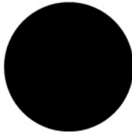
Gambar 1: Sebuah kulit bola yang menggambarkan seekor sapi.
