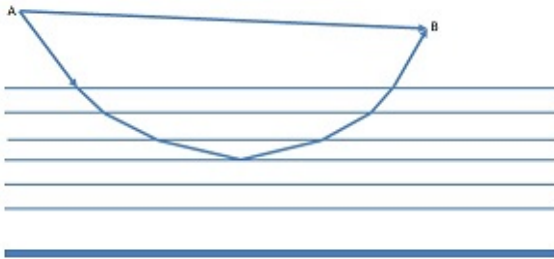
Gambar 8: Gerak cahaya sampai ke mata saat terjadi fatamorgana.
