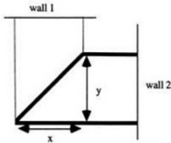
Gambar 28: Penggaris yang diputar akan memiliki panjang proyeksi yang berbeda.
