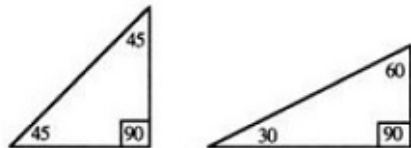
Gambar 33: Konsep sudut dalam segitiga.
