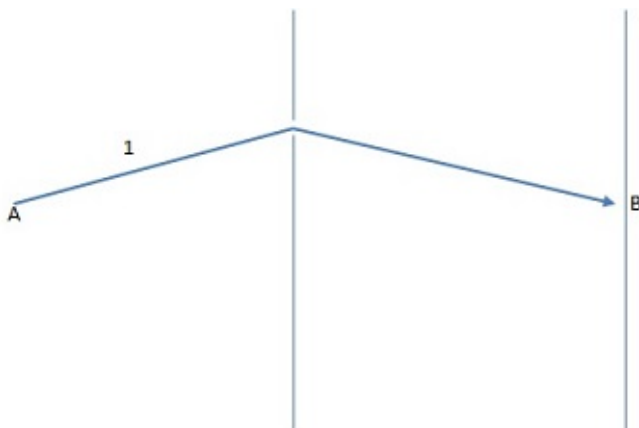
Gambar 11: Jalur yang dilalui oleh partikel dari A ke B.
