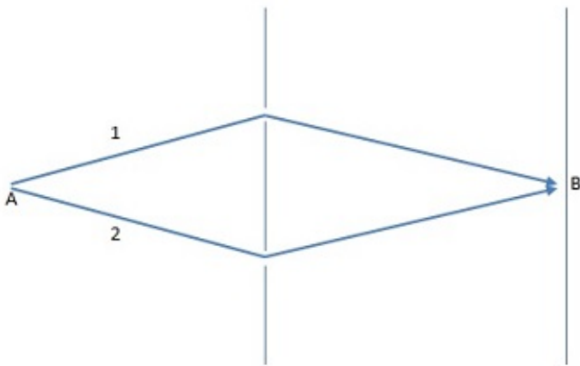
Gambar 13: Probabilitas partikel yang melalui dua jalur yang diizinkan dapat memiliki ‘probabilitas’ nol.
