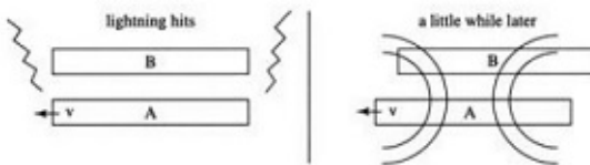
Gambar 24: Kejadian yang diamati oleh B.
