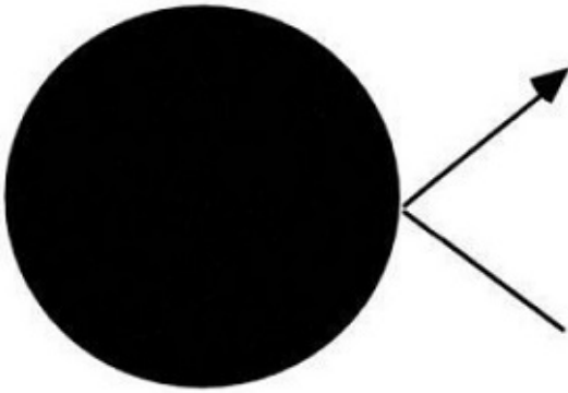
Gambar 45: Prediksi pantulan hasil lemparan.
