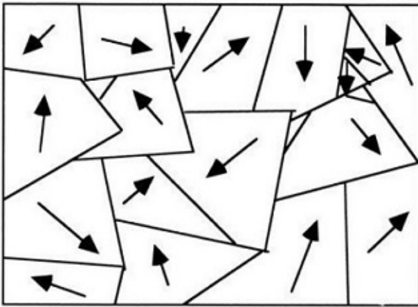
Gambar 44: Materi yang tidak dibatasi untuk menunjuk naik dan turun seperti magnet mikroskopis.
