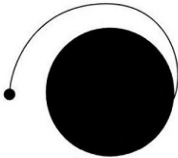
Gambar 31: Proyeksi dua dimensi dari gerak sebuah benda.
