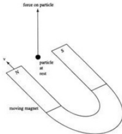
Gambar 20: Arah gaya pada partikel saat bergerak bersama dengan partikel dengan kecepatan konstan.
