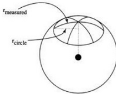
Gambar 35: Melihat kulit bola dari luar.
