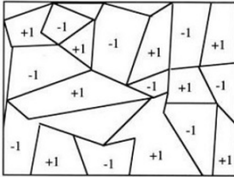
Gambar 39: Gambaran kepadatan atau densitas pada titik kritis.
