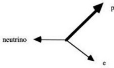
Gambar 42: Munculnya konsep neutrino salah satunya adalah untuk mempertahankan konsep kelestarian momentum (dan juga energi).
