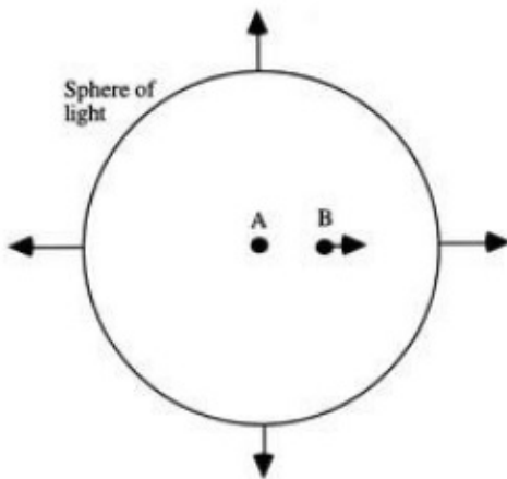
Gambar 21: Pengamat A diam terhadap bola lampu.
