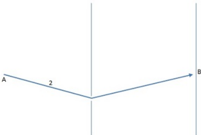
Gambar 12: Jalur lain yang dilalui oleh partikel dari A ke B.
