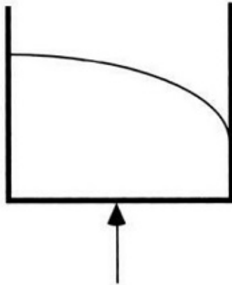
Gambar 29: Jalur sinar cahaya akan tampak seperti ini di dalam lift yang dipercepat.
