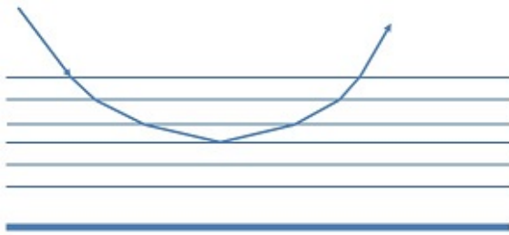
Gambar 7: Pembelokkan sinar pada lapisan kepadatan medium saat terjadi fatamorgana.
