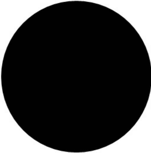
Gambar 2: Sebuah kulit bola yang lebih besar menggambarkan sapi-super yang identik dengan penggambaran seekor sapi normal.
