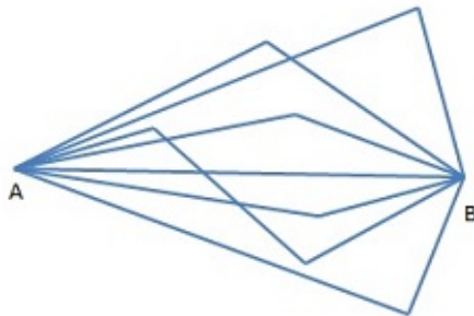
Gambar 10: Jalur yang mungkin dilalui oleh partikel dari titik A ke titik B.
