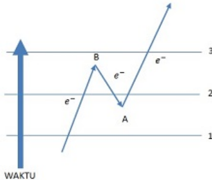
Gambar 14: Gambaran lompatan waktu.
