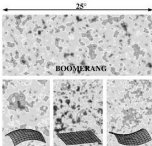
Gambar 38: Geometri alam semesta datar.
