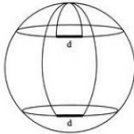
Gambar 37: Penurunan sudut tinjauan tidak akan terjadi jika pada kulit bola.
