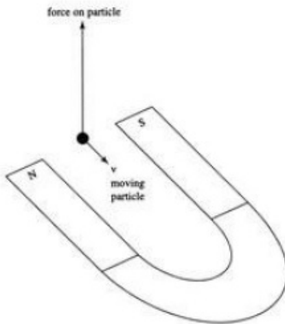
Gambar 19: Arah gaya pada partikel saat partikel bermuatan bergerak secara horizontal di antara kutub magnet.
