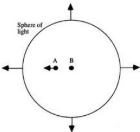
Gambar 22: A telah pindah ke kiri pusat.
