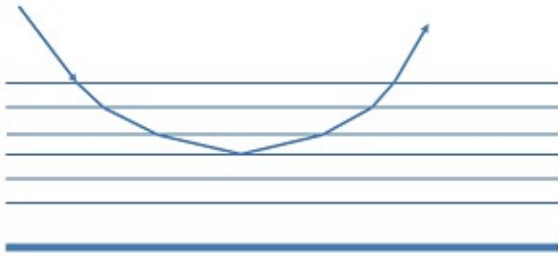
Gambar 7: Pembelokkan sinar pada lapisan kepadatan medium saat terjadi fatamorgana.
