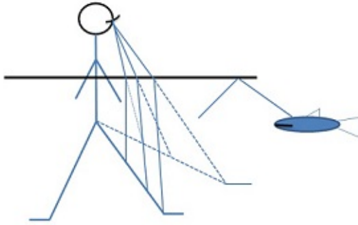
Gambar 6: Sinar cahaya membengkok pada permukaan dan menge- labui seseorang dengan berpikir kaki Anda lebih tinggi dari mereka.
