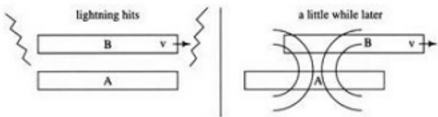
Gambar 23: Sambaran petir di depan dan di belakang kereta.
