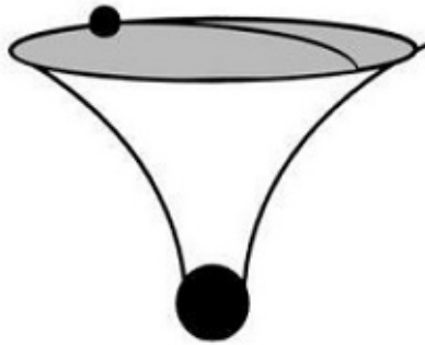
Gambar 32: Objek tidak merasakan gaya yang diberikan oleh bola besar.
