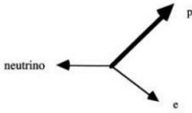
Gambar 42: Munculnya konsep neutrino salah satunya adalah untuk mempertahankan konsep kelestarian momentum (dan juga energi).
