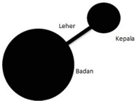
Gambar 4: Sapi dengan dua kulit bola (dihubungkan dengan sebuah batang).
