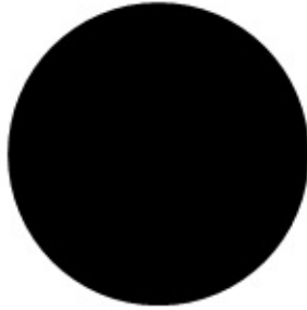
Gambar 17: Pada Senin malam gambar menjadi berbentuk cakram.
