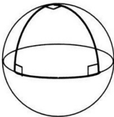
Gambar 34: Segitiga pada permukaan kulit bola.
