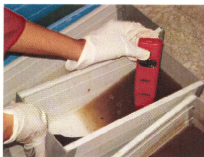
Pengukuran pH cairan rendaman dengan pH meter digital
