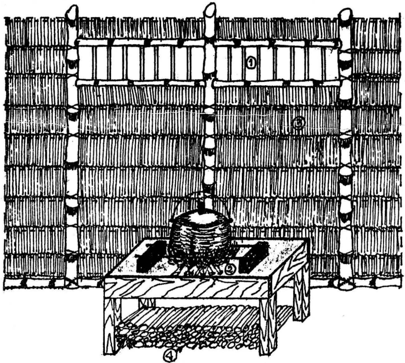
Gambar No. : 7. Dinding dapur dibahagian tungku masak model berdiri.
